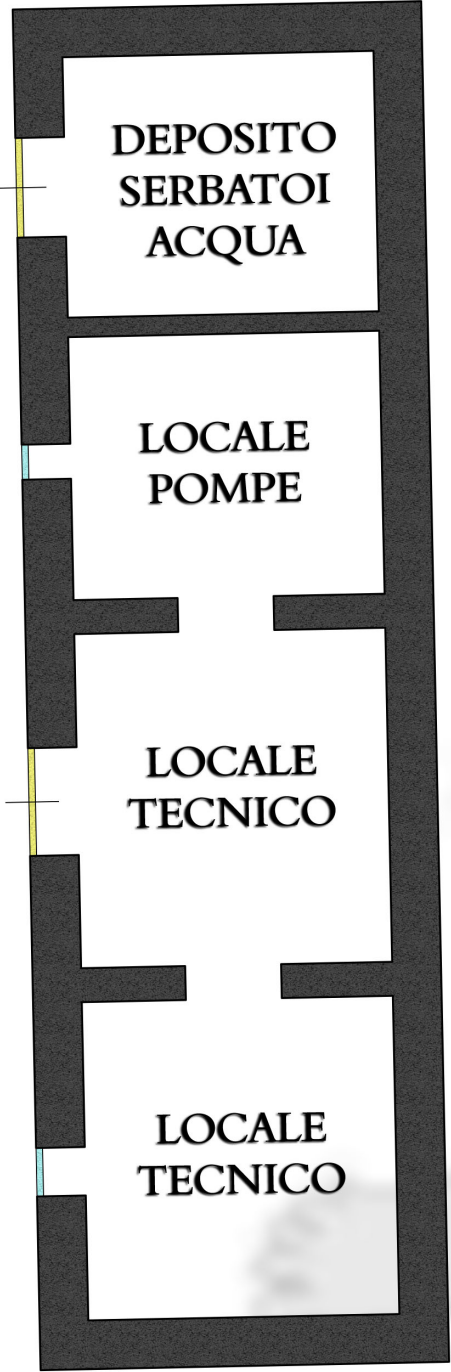
EDIFICIO TECNICO
