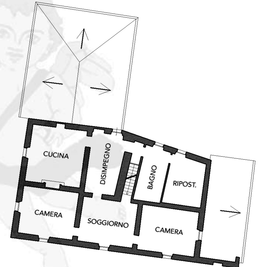
PIANO SECONDO
