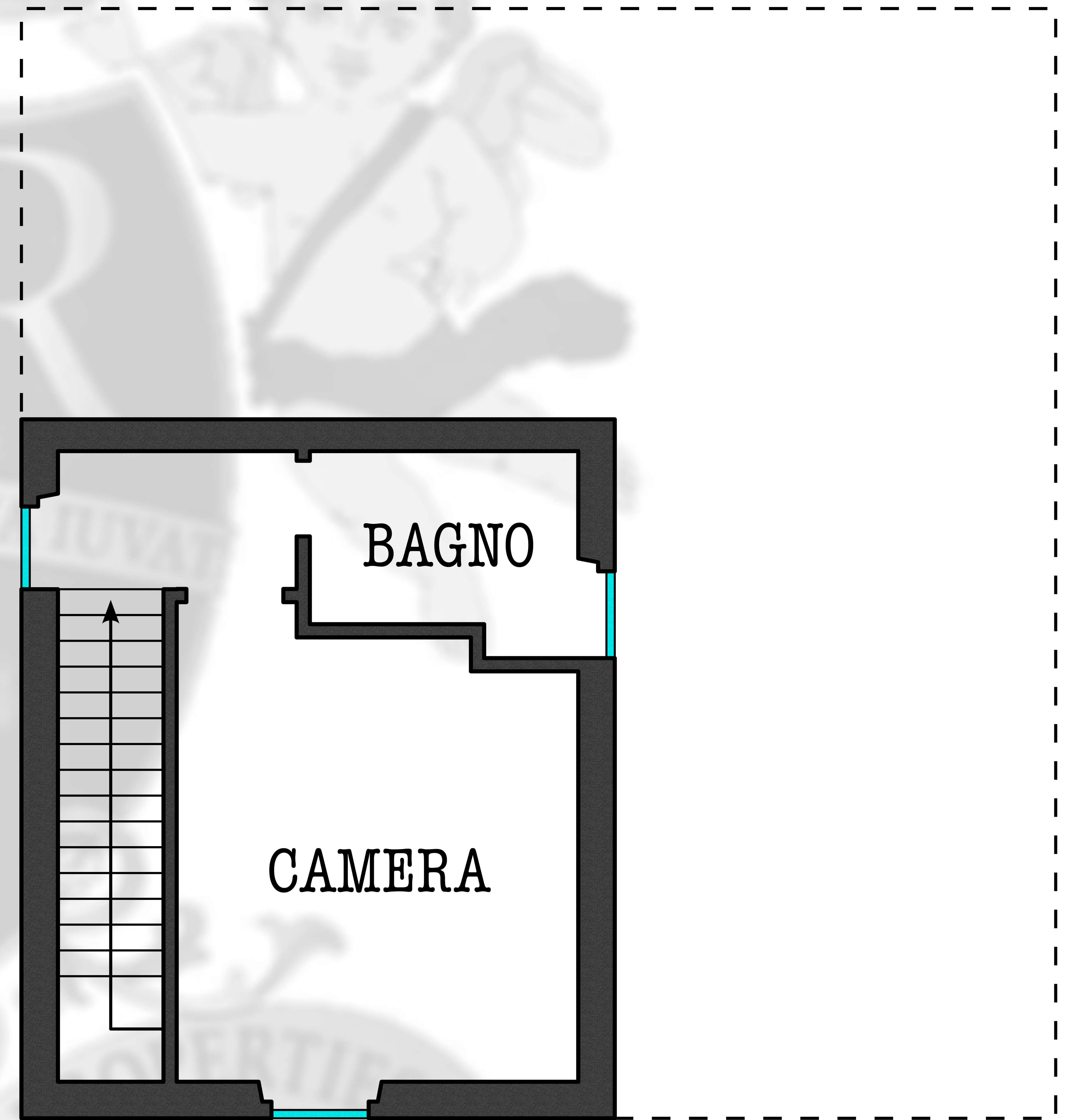
PIANO PRIMO
